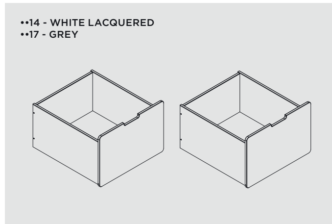
PILD90•• W 558 mm - H 396 mm - D 600 mm
