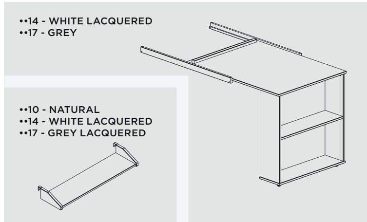
PIOLHP•• W 793 mm - H 90 mm - D 210 mm
